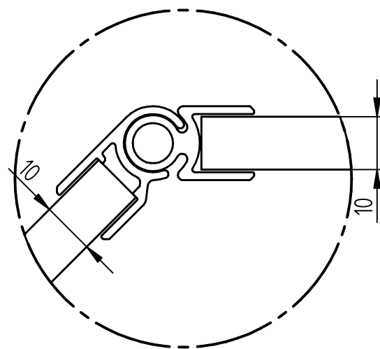
EINZELHEIT A
